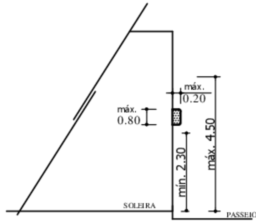
CORTE ESQUEMATICO
